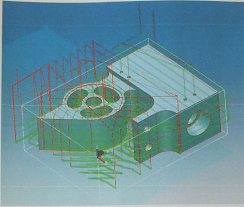
Obrázek 69 Dráhy nástroje při prvním nastavení součásti
