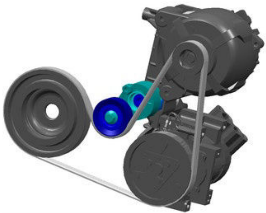
Mechanický napínák emenu
